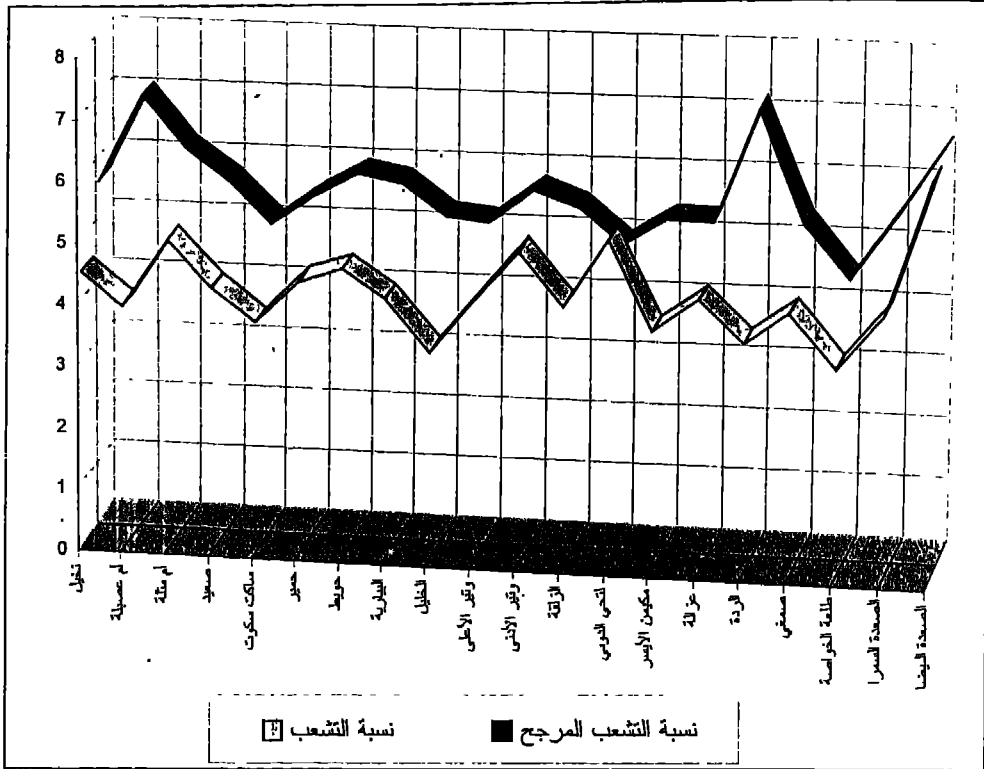
شكل (٣-٥) العلاقة بين نسبة التشعب ونسبة التشعب المرجح لأحواض الروافد
