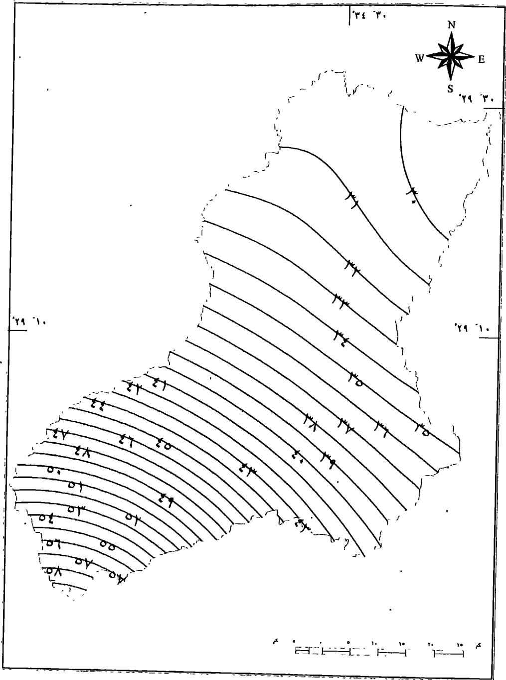
شكل (٢-٤) خطوط المطر المتساوي لحوض وادي وتير (بالمليمت)
