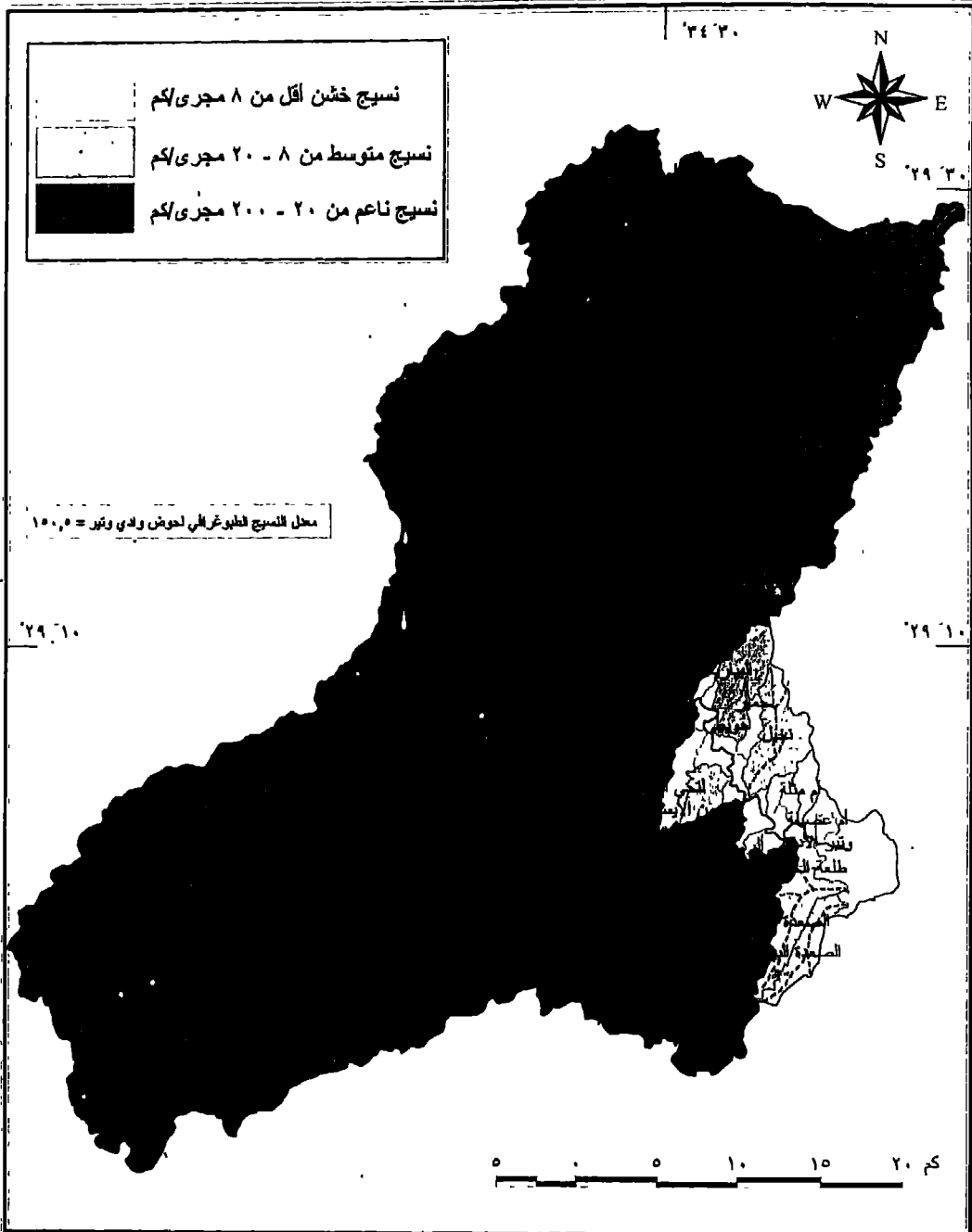
شكل (٣-١٦) معدل النسيج الطبوغرافي في حوض وادي وتير وروافده
