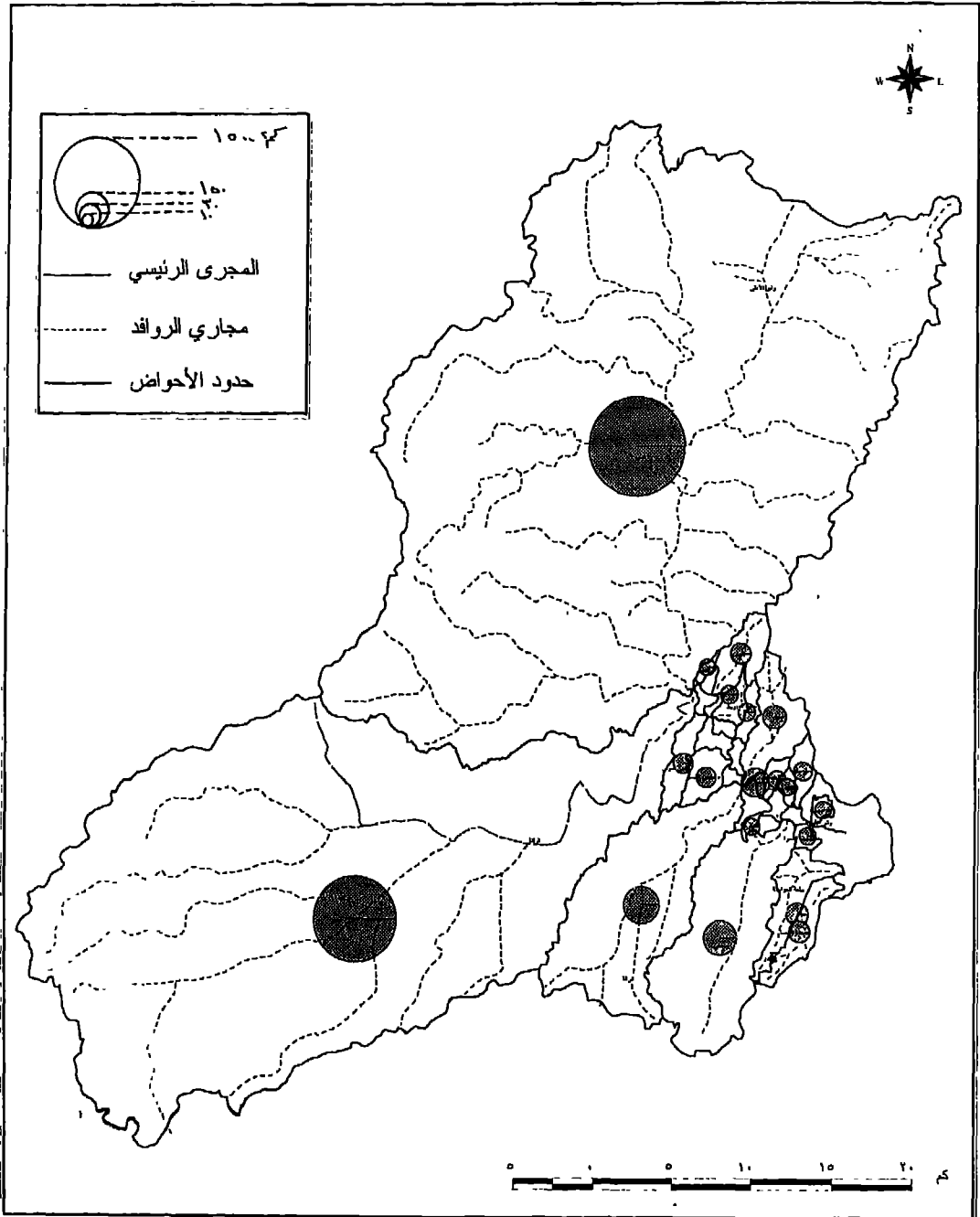
تصنيف الأودية حسب مساحتها
