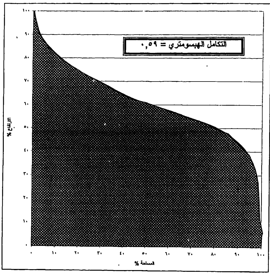
شكل (٢-١٦) المنحنى الهيسومتري لحوض وادي وتير
