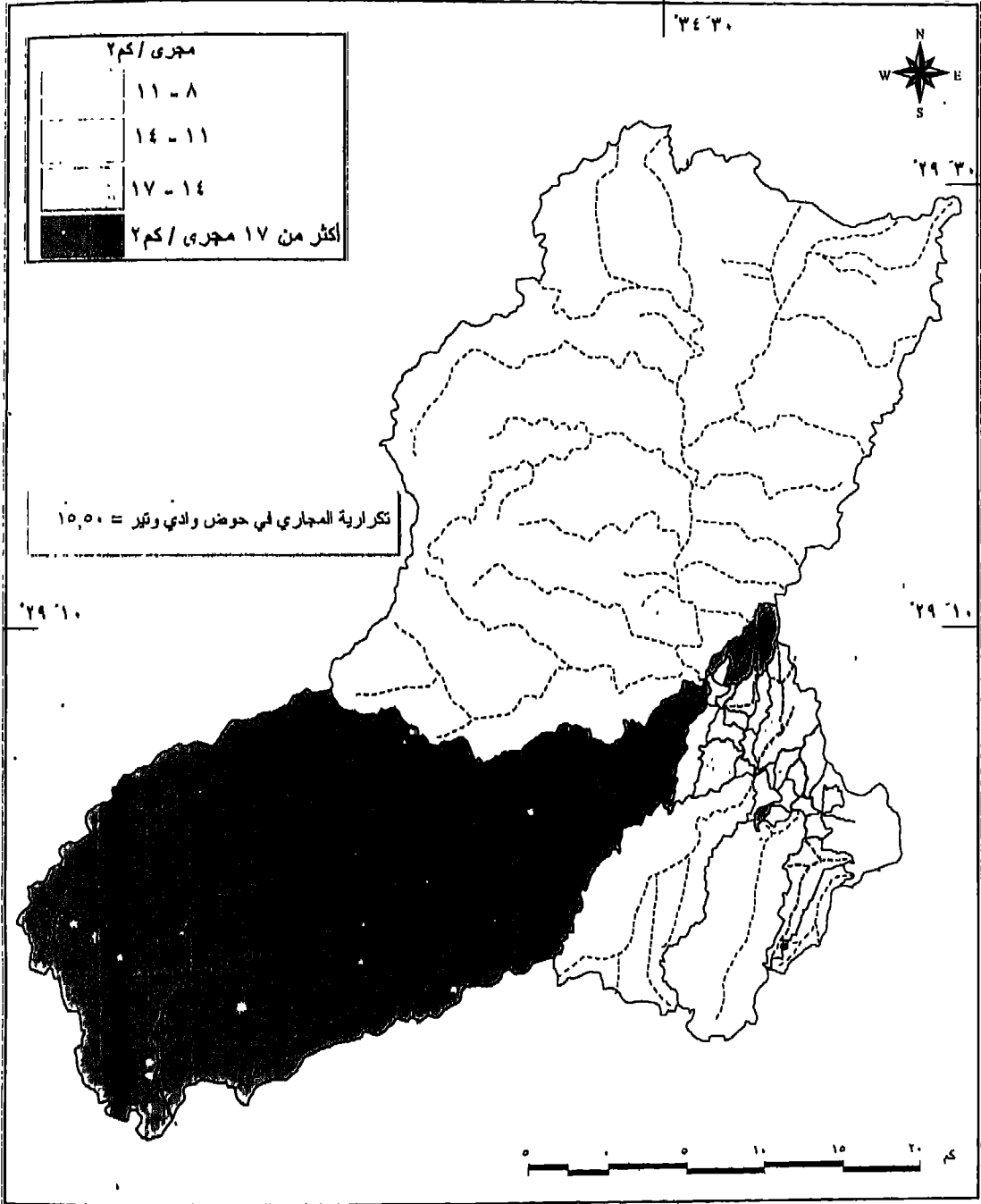
تكرارية المجاري في حوض وادي وتير وروافده
