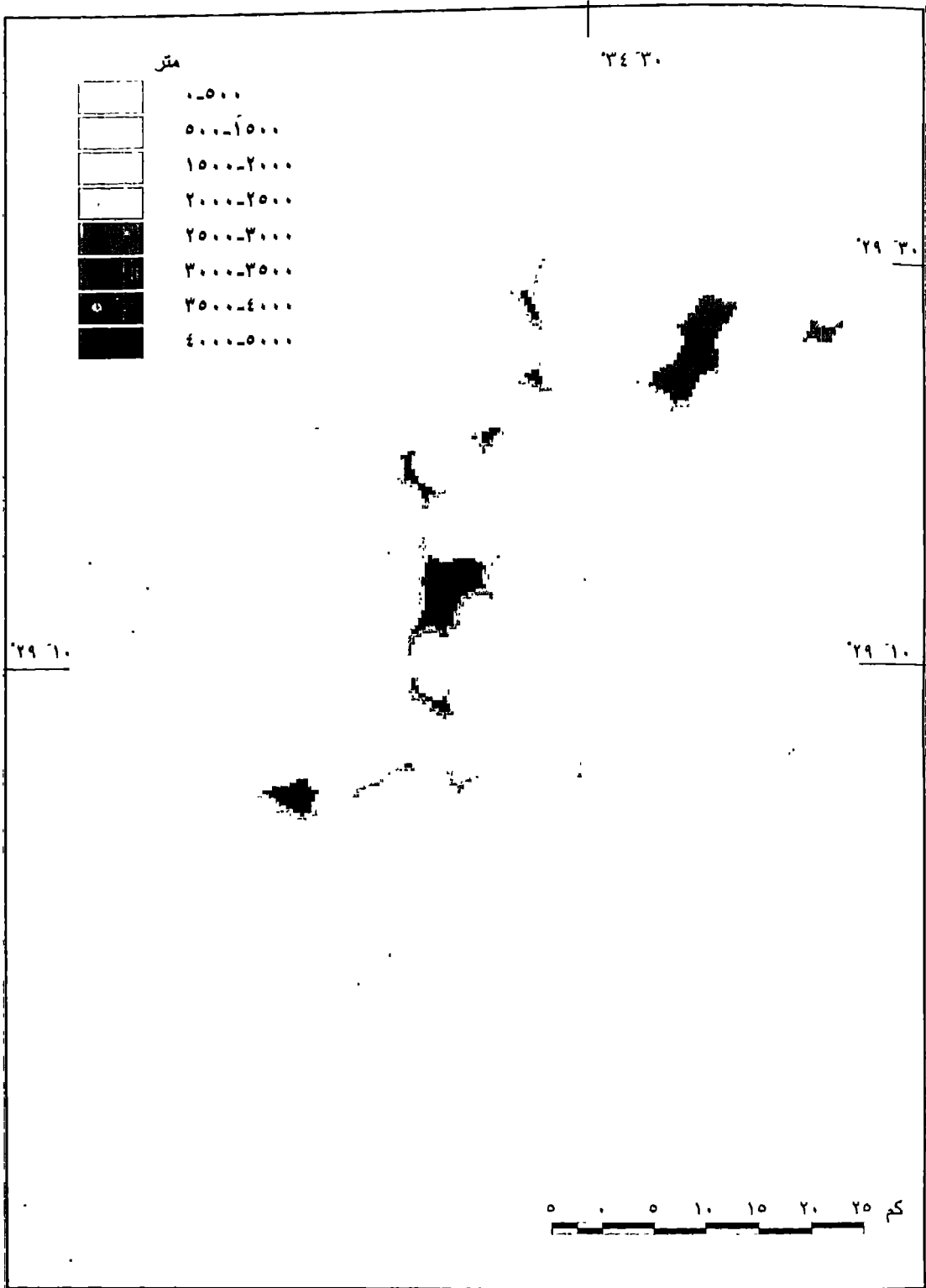
شکل (٢-١٢) المسافات بين خطوط الكنتور في حوض وادي وتير
