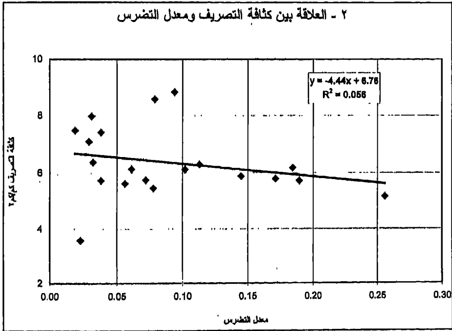
شكل (٣-١٩) العلاقة بين كثافة التصريف وكل من المساحة ومعدل التضرس
