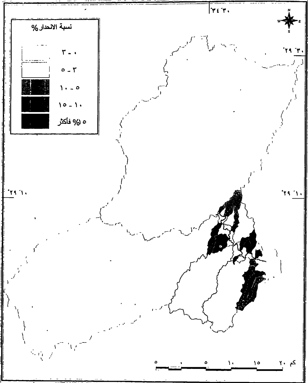
شكل (١٥-٢) نسب الانحدار في أحواض الروافد الرئيسية
