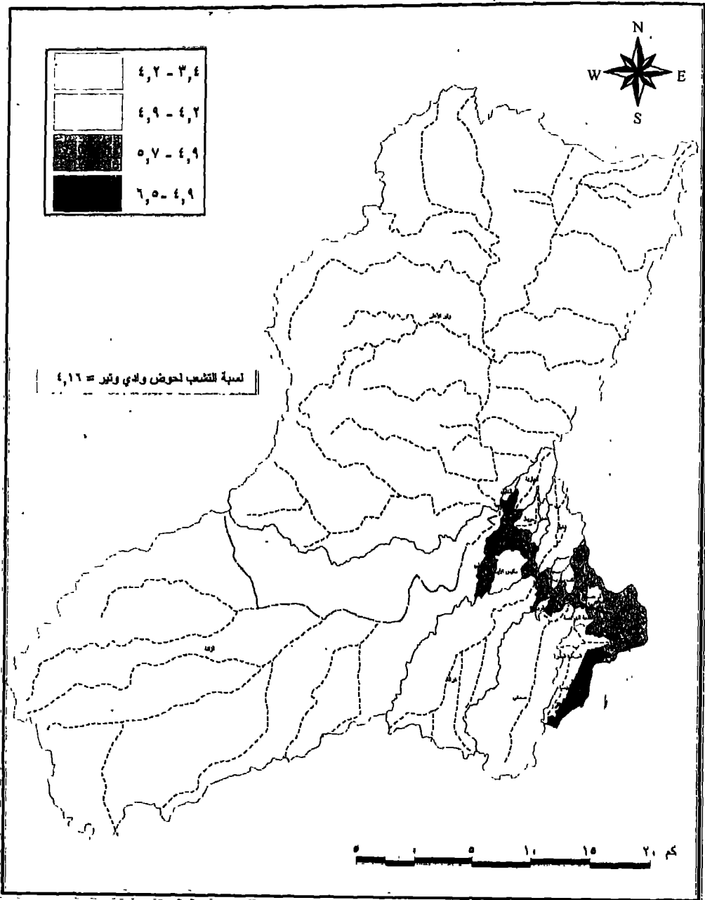
شكل (٤-٣) نسبة التشعب في حوض وادي وثير وروافده
