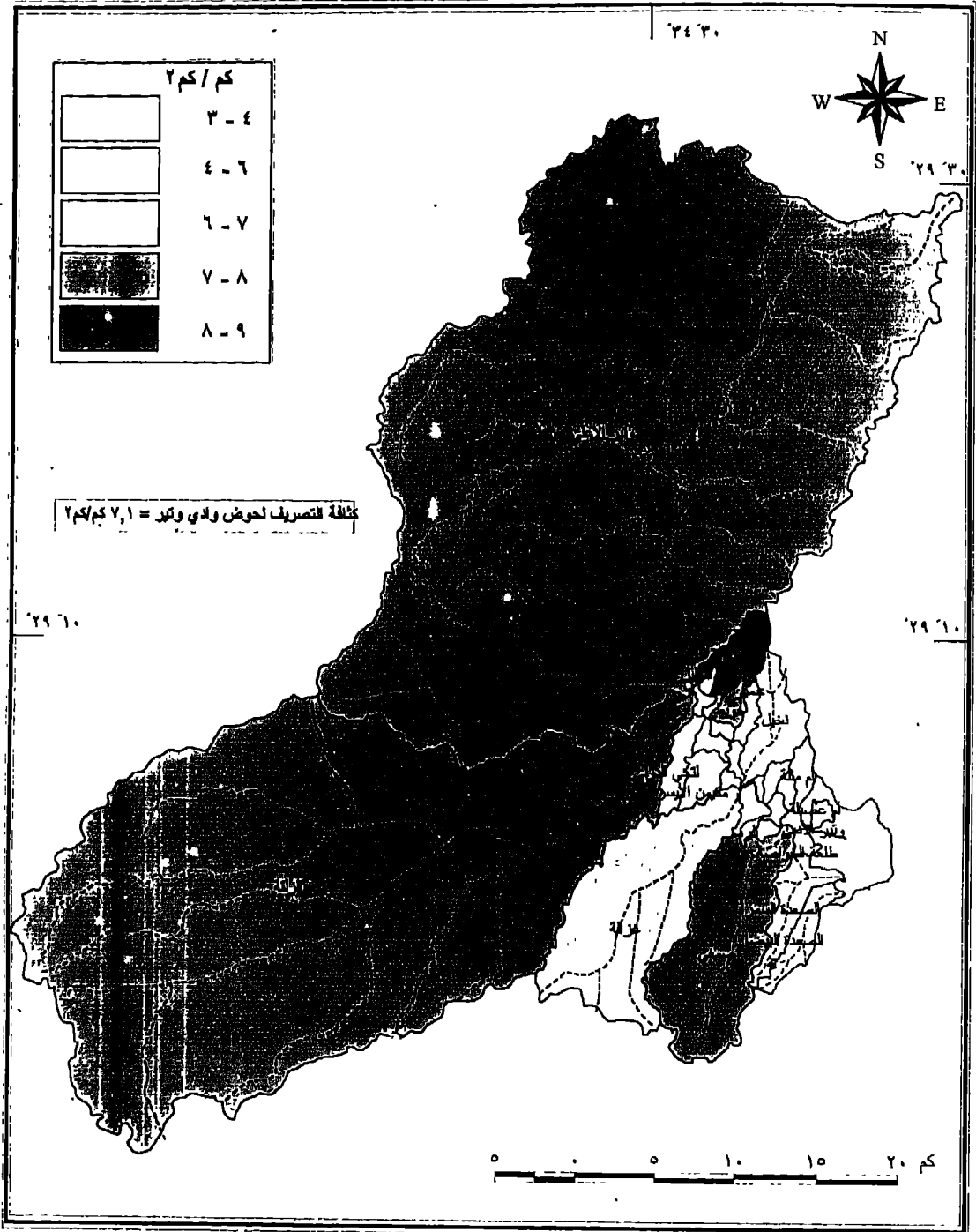
كثافة التصريف في حوض وادي وتير
