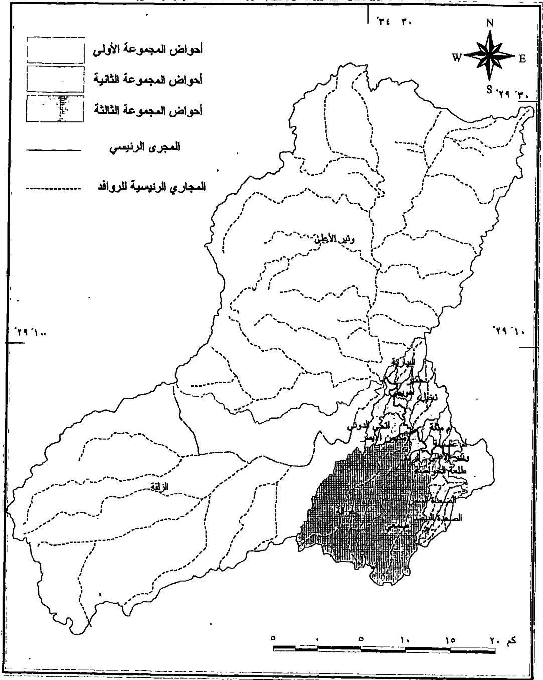
شكل (٣-٢٣) التحليل العقودي لمتغيرات الأحواض والشبكات
