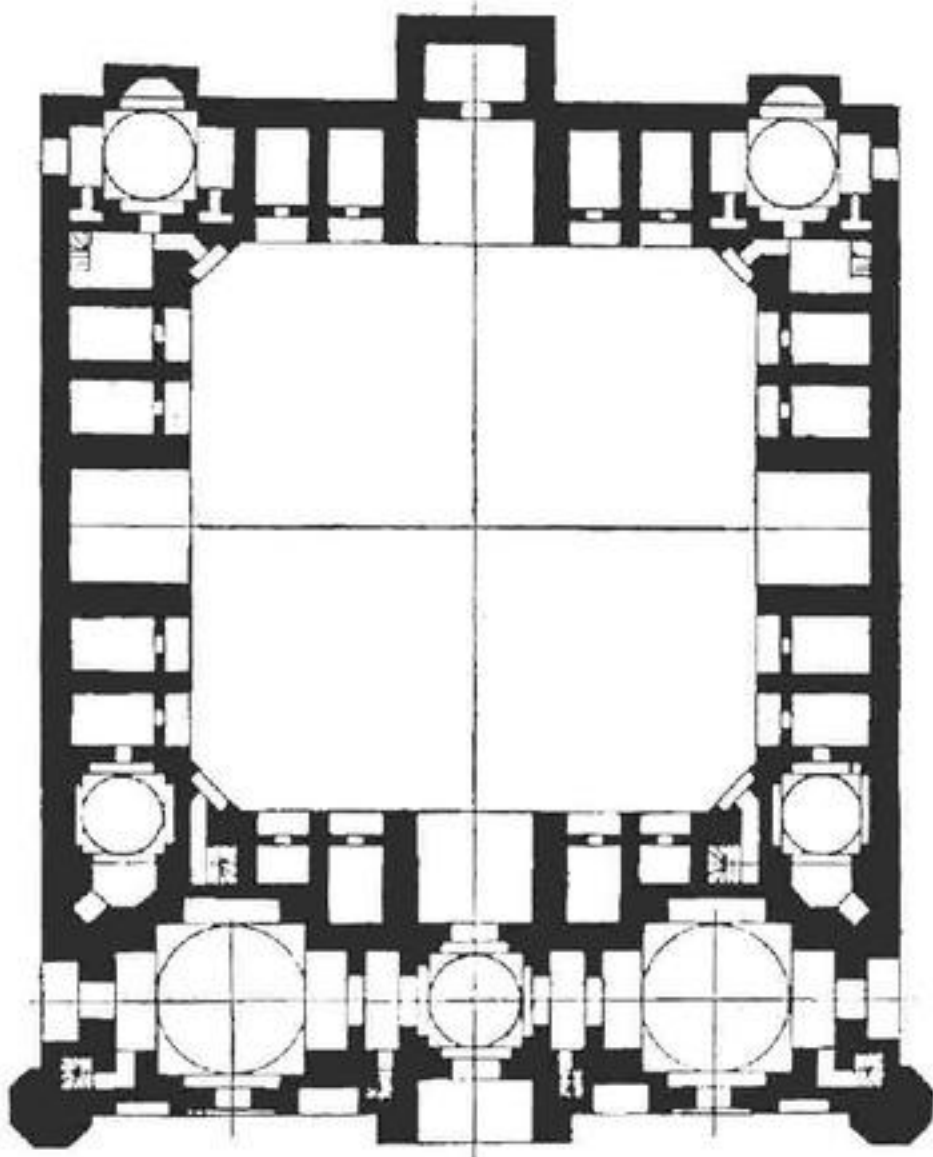
(شكل ٢٩) تخطيط مدرسة خربد
